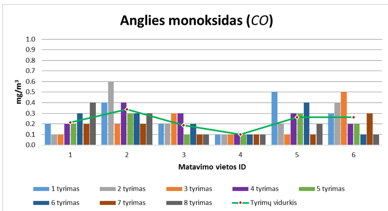
16 pav. Anglies monoksido koncentracijų pasiskirstymai Druskininkuose pagal nustatytos matavimo vietos ID. (Ribinė vertė 10 \text{ mg}/\text{m}^3 grafike neatvaizduojama, nes gautos CO koncentracijų vertės ženkliai mažesnės)
