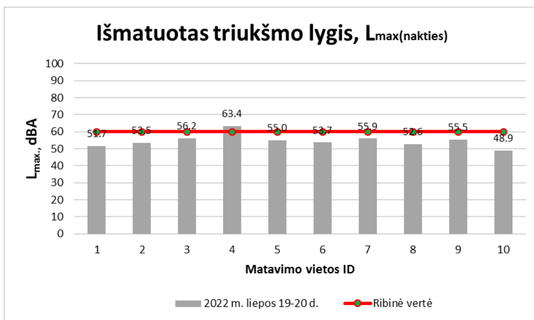
39 pav. Maksimalaus triukšmo pasiskirstymas matavimo vietose nakties metu (22-7 val.). Ribinis dydis 60 dBA
