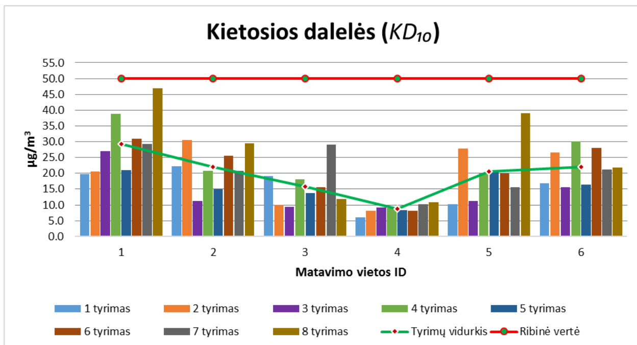
15 pav. Kietųjų dalelių koncentracijų pasiskirstymai Druskininkuose pagal nustatytos matavimo vietos ID.
