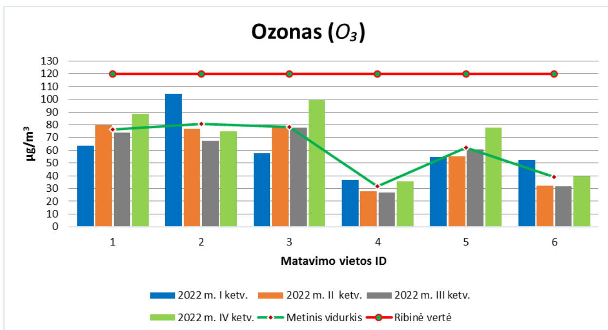
14 pav. Ozono koncentracijų pasiskirstymai Druskininkuose pagal nustatytos matavimo vietos ID.
