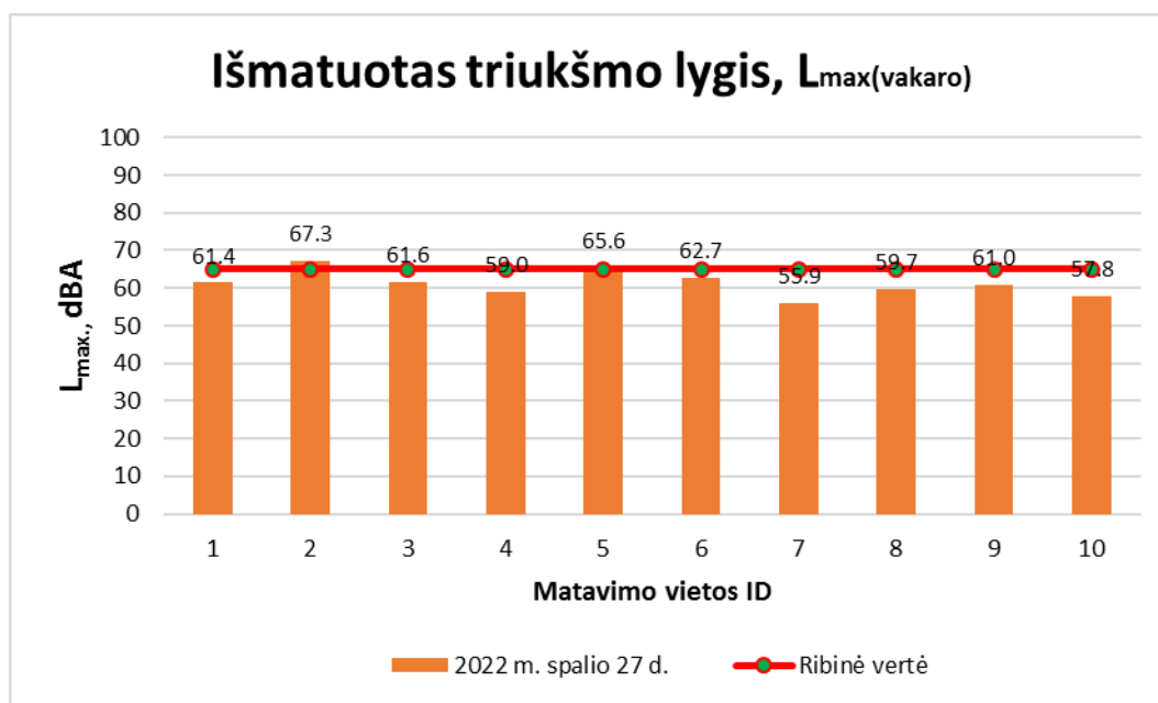
45 pav. Maksimalaus triukšmo pasiskirstymas matavimo vietose vakaro metu (19-22 val.). Ribinis dydis 65 dBA
