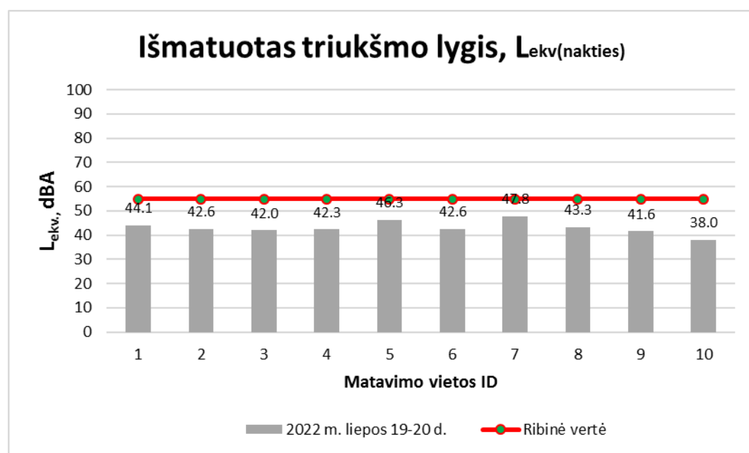
40 pav. Ekvivalentinio triukšmo pasiskirstymas matavimo vietose nakties metu (22-7 val.). Ribinis dydis 55 dBA
