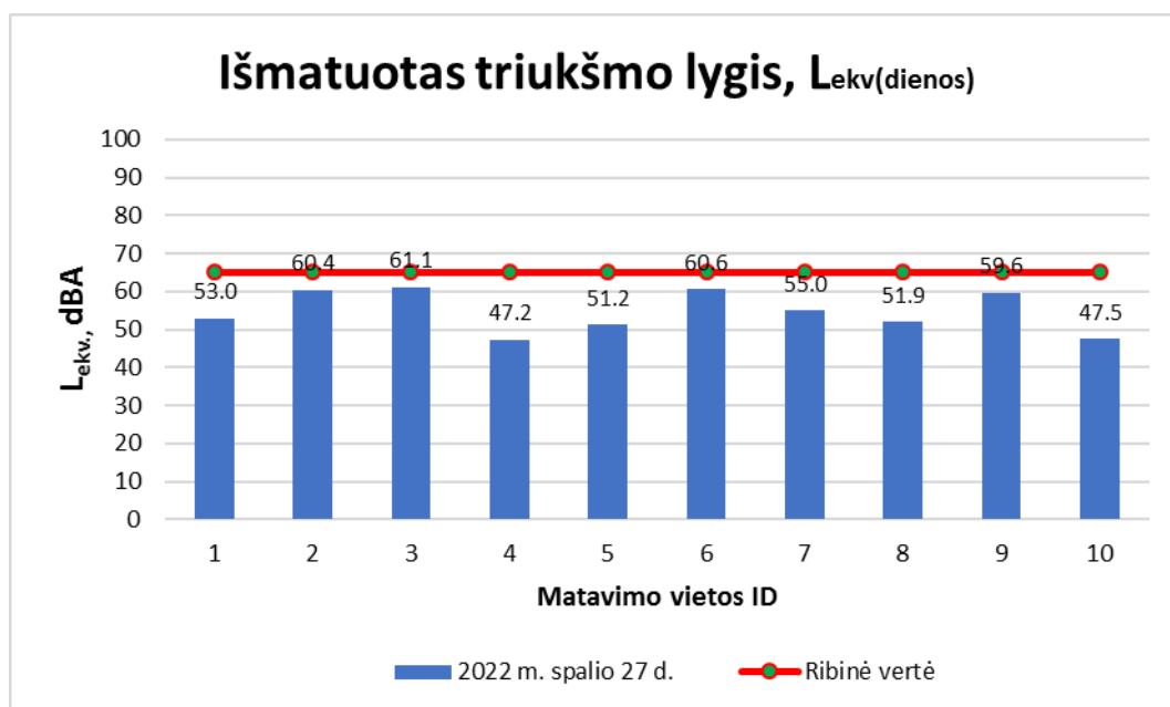
44 pav. Ekvivalentinio triukšmo pasiskirstymas matavimo vietose dienos metu (7-19 val.).
