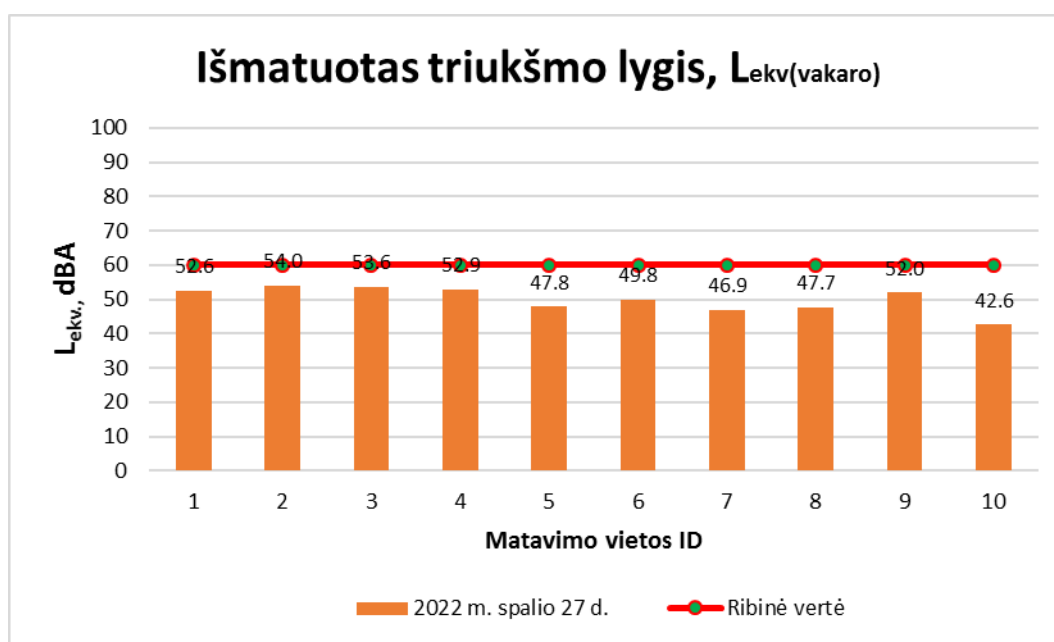
46 pav. Ekvivalentinio triukšmo pasiskirstymas matavimo vietose vakaro metu (19-22 val.). Ribinis dydis 60 dBA
