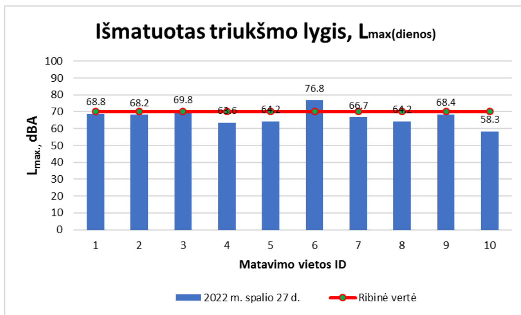
43 pav. Maksimalaus triukšmo lygio pasiskirstymas matavimo vietose dienos metu (7-19 val.).
