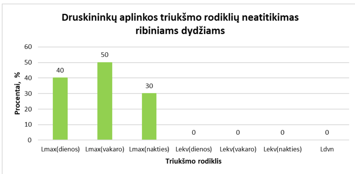
20 pav. Triukšmo matavimo vietų, kuriose viršijami ribiniai dydžiai, skaičius procentais
