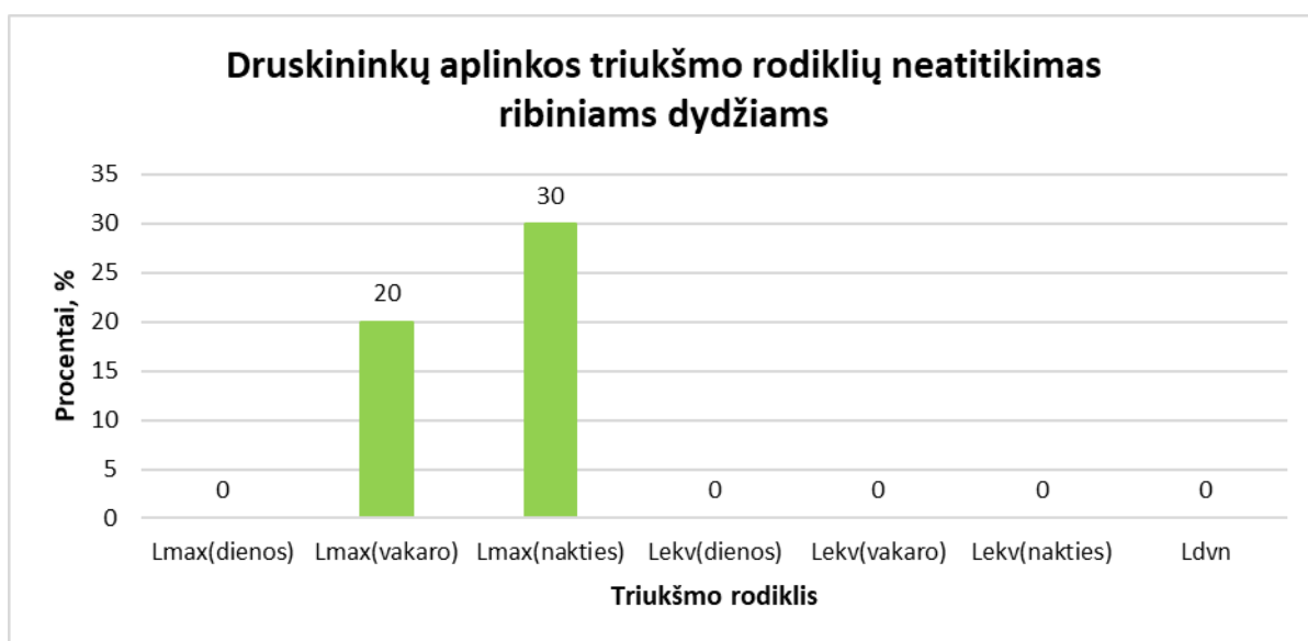
44 pav. Triukšmo matavimo vietų, kuriose viršijami ribiniai dydžiai, skaičius procentais.
