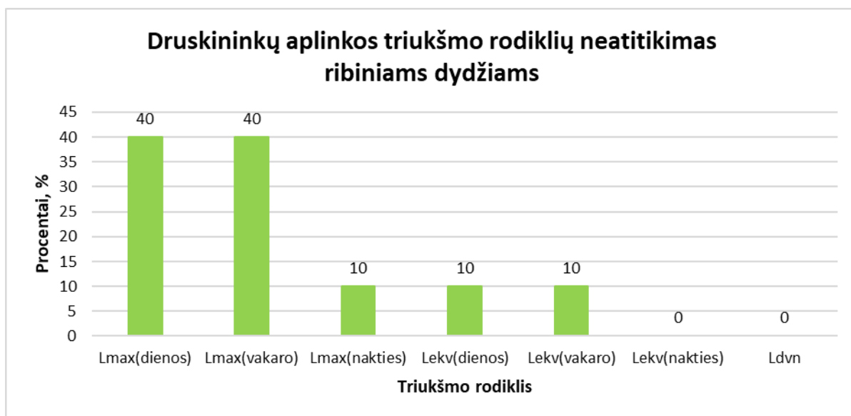
28 pav. Triukšmo matavimo vietų, kuriose viršijami ribiniai dydžiai, skaičius procentais.
