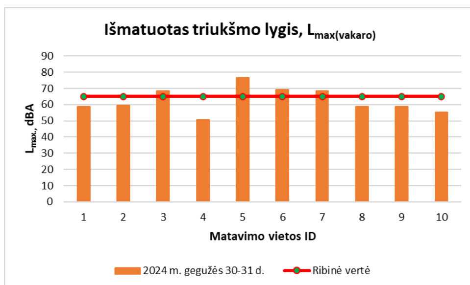
23 pav. Maksimalaus triukšmo pasiskirstymas matavimo vietose vakaro metu (19 – 22 val.).
