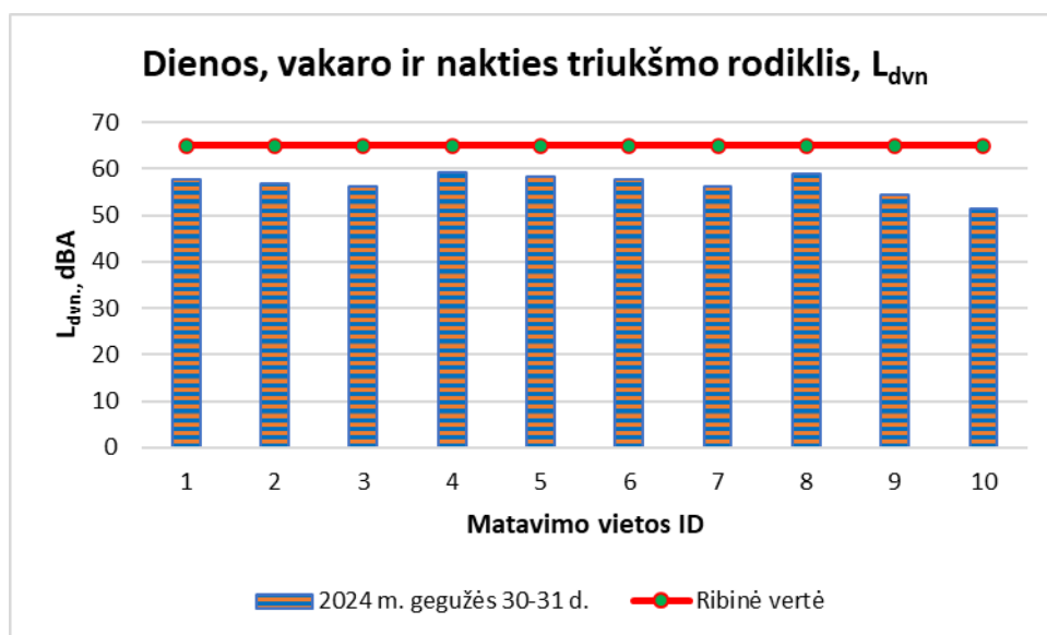
27 pav. Dienos, vakaro ir nakties triukšmo rodiklio ( L_{\text{dvn}} ) pasiskirstymas matavimo vietose. Ribinis dydis 65 dBA
