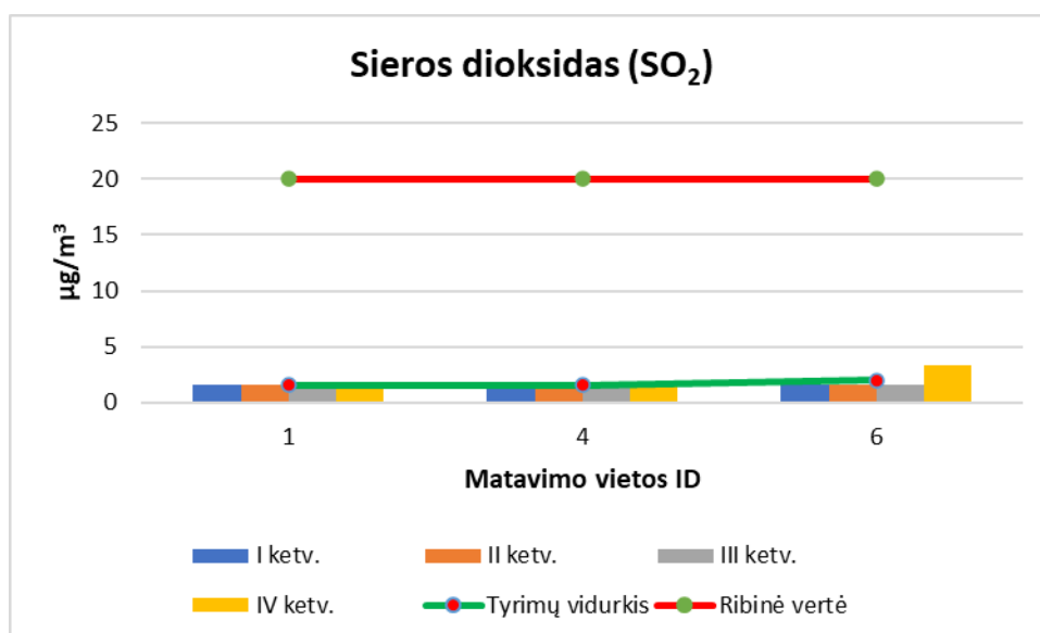
6 pav. SO 2 koncentracijų pasiskirstymas Druskininkuose, nustatytose matavimų vietose
