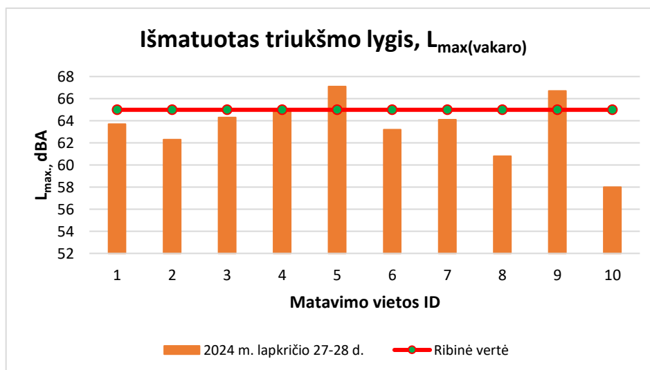
39 pav. Maksimalaus triukšmo pasiskirstymas matavimo vietose vakaro metu (19 – 22 val.). Ribinis dydis 65 dBA
