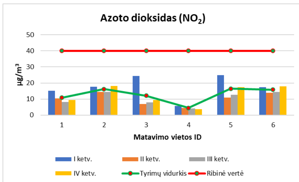
5 pav. NO 2 koncentracijų pasiskirstymas Druskininkuose, nustatytose matavimų vietose
