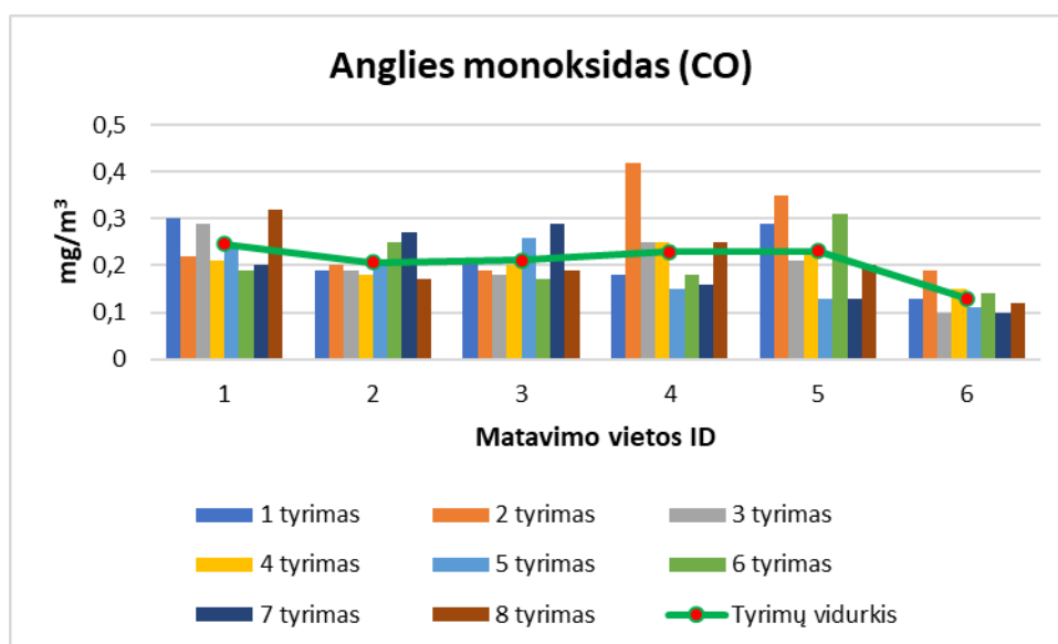
10 pav. Anglies monoksido koncentracijų pasiskirstymai Druskininkuose pagal nustatytos matavimo vietos ID. (Ribinė vertė 10 \text{ mg}/\text{m}^3 grafike neatvaizduojama, nes gautos CO koncentracijų vertės ženkliai mažesnės)
