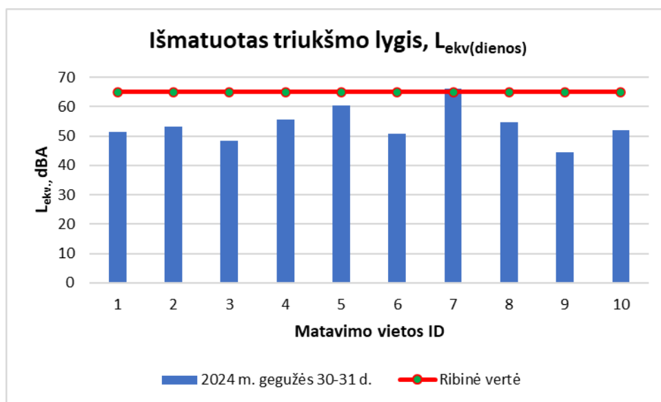
22 pav. Ekvivalentinio triukšmo pasiskirstymas matavimo vietose dienos metu (7 – 19 val.).
