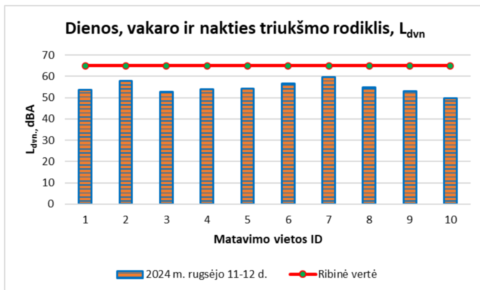
35 pav. Dienos, vakaro ir nakties triukšmo rodiklio ( L_{dvn} ) pasiskirstymas matavimo vietose.
