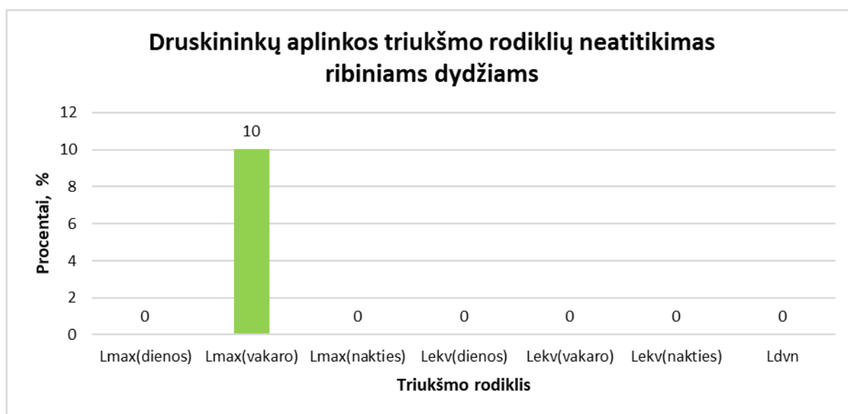
36 pav. Triukšmo matavimo vietų, kuriose viršijami ribiniai dydžiai, skaičius procentais.
