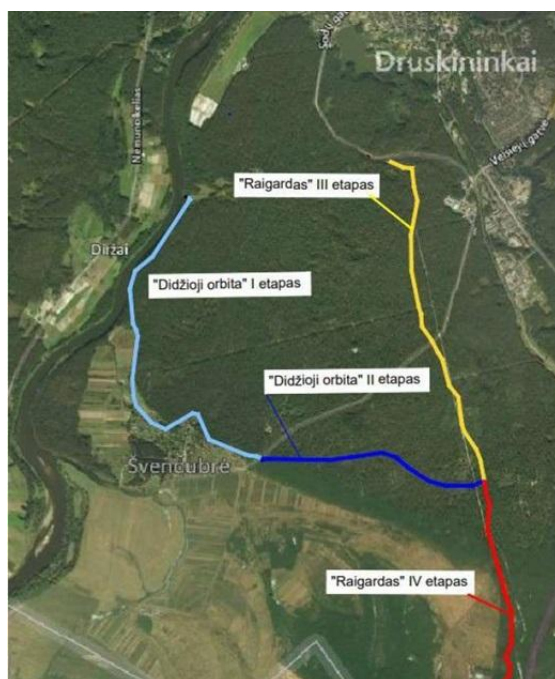
pav. 39. Dviračių tako „Žvaigždžių orbita“ schema
