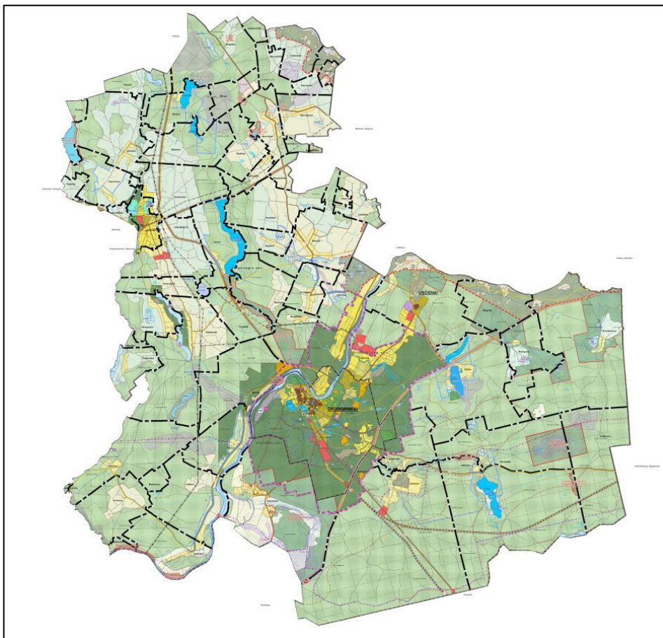
Pav. 73. Druskininkų savivaldybės teritorijos bendrojo plano pagrindinis brėžinys
