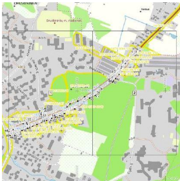
Pav. 74. Neravų gatvės, Druskininkuose, sprendinių brėžinys
